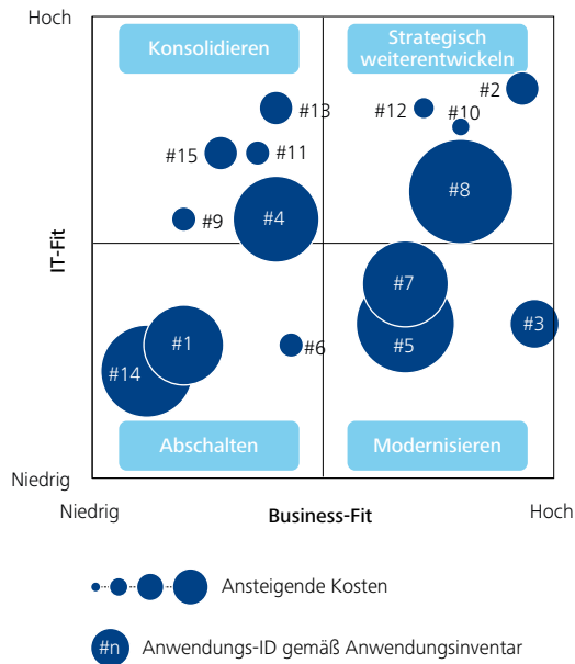
Abb. 2 – APR Bewertungsmatrix
