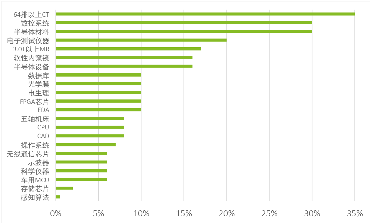
图 8 2021 年科技制造领域关键设备、系统国产化率
